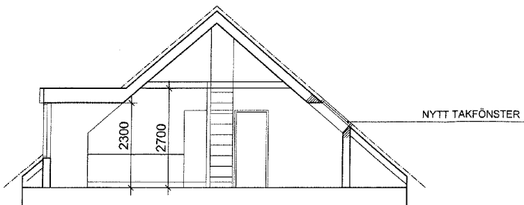
SEKTION A-A
