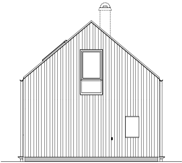
FASAD D
